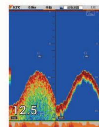
魚探2周波画面
